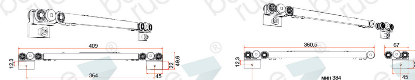
Механизм раздвижения с двухсторонним доводчиком для полотен 430–600 мм Механизм раздвижения с двухсторонним доводчиком для полотен 450–1100 мм
